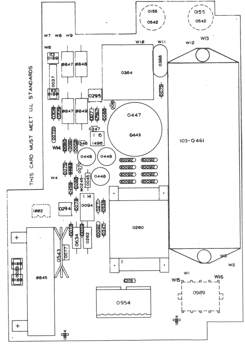
00300098502 LAYER 3
