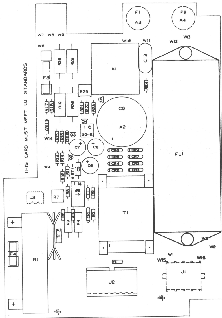
00300098502 LAYER 5
