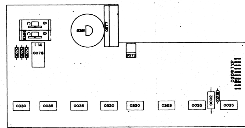
00300092205 LAYER 5
