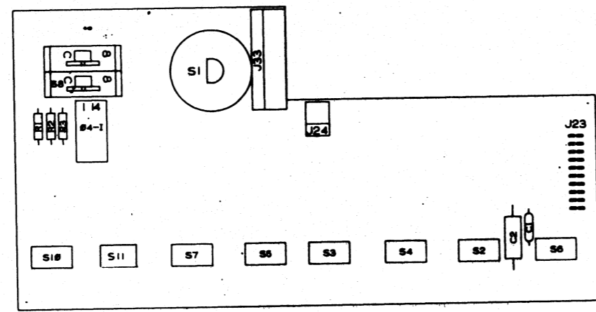
00300092205 LAYER 6
